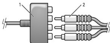
1 元件影像配接卡 2 元件影像纜線
