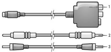
1 合成式影像配接卡 2 合成式影像纜線 3 標準音效纜線
